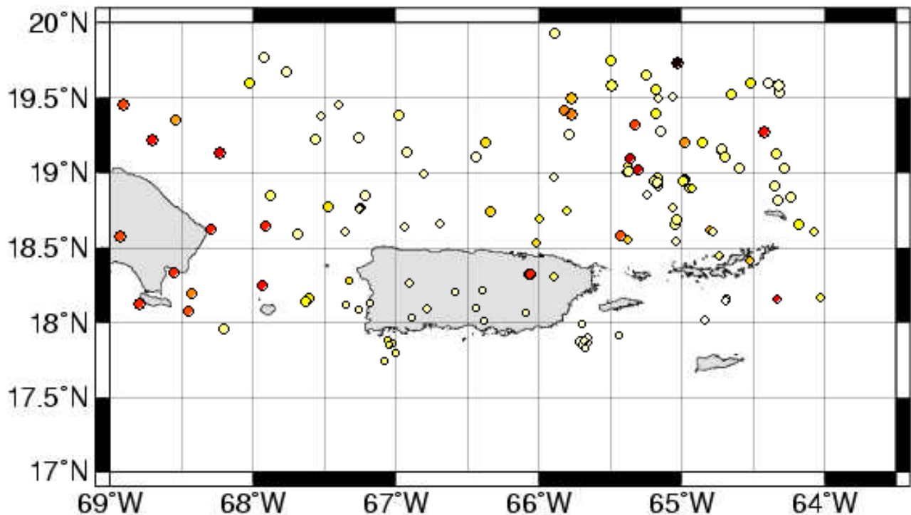
Figura 1. Mapa epicentral de los sismos localizados por la RSPR para el mes de agosto de 2008 (RSPR-UPRM).
