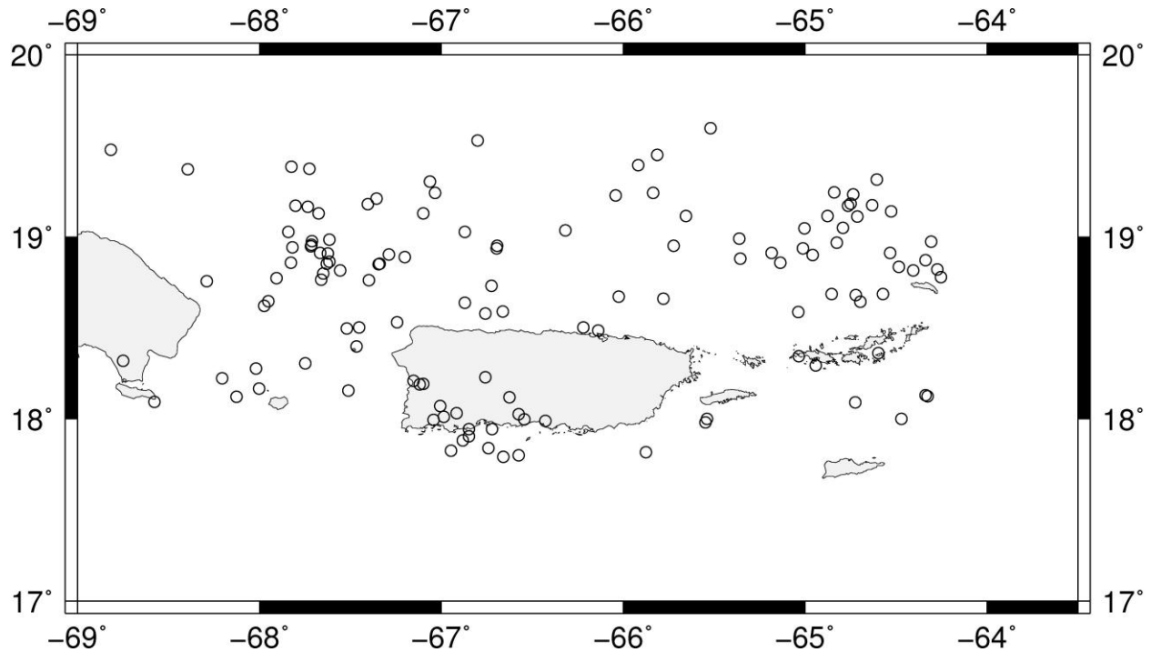
Figura 1. Mapa epicentral de los sismos localizados por la RSPR para el mes de octubre de 2011 (RSPR-UPRM).
